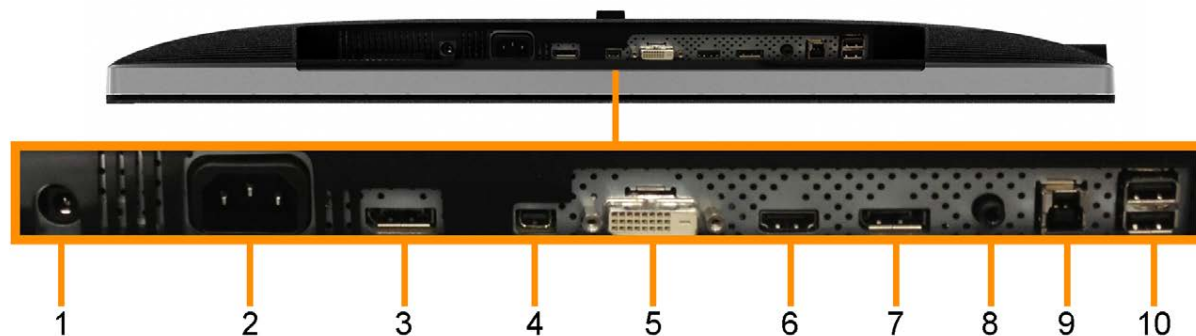
無顯示器支架的底視圖
